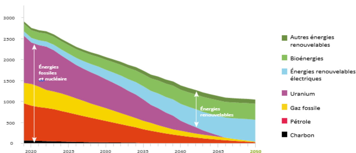
Fig 6 : Evaluation de la consommation d'énergie primaire pour les usages énergétiques et les usages matières dans le scénario négaWatt entre 2019 et 2022
