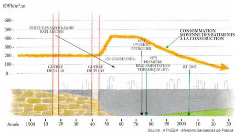
Fig 5 : Evolution de la consommation moyenne des bâtiments à la construction à partir de 1900
